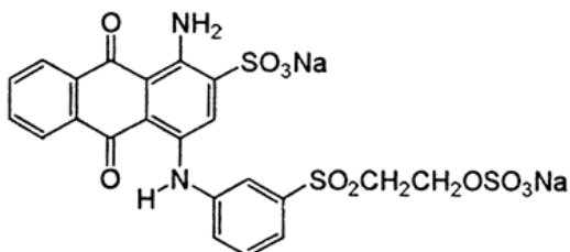
Colorante reactivo con grupo reactivo vinilsulfona (C.I. Reactive Blue 19)
