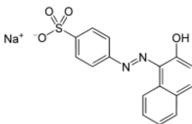
Estructura química de un colorante azoico (C.I. Acid Orange 7, Numero C.I 15510)
